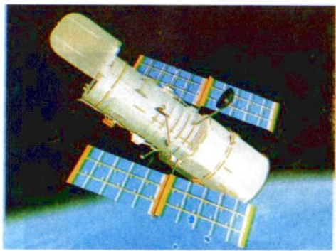
Американский телескоп Хаббла
